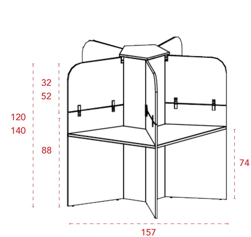
Call center acústico / isla de 5 puestos / curvo.
