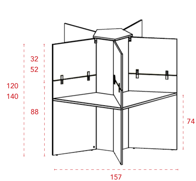
Call center acústico / isla de 5 puestos / recto.
